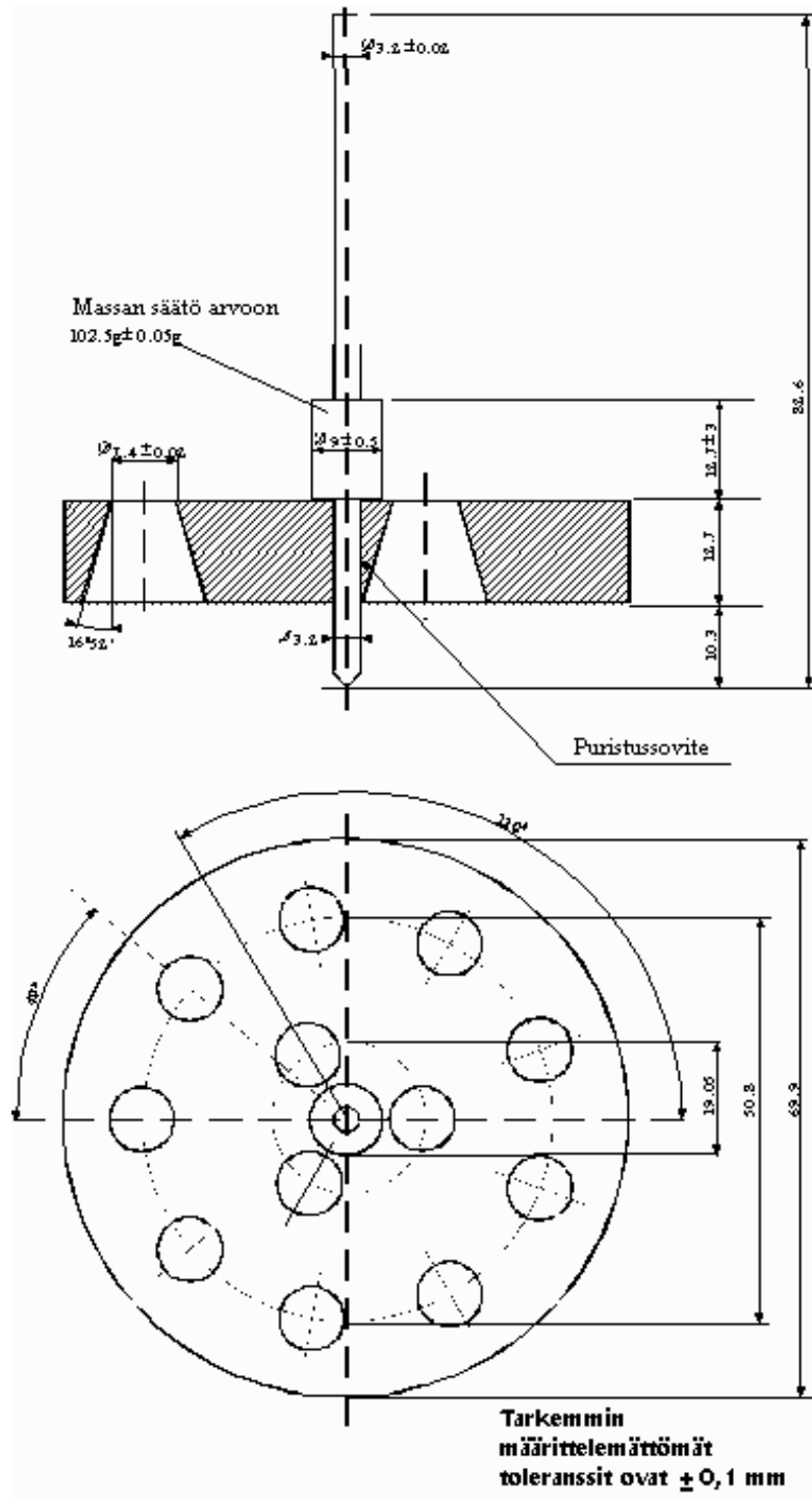
Kuva 1: Penetrometri
