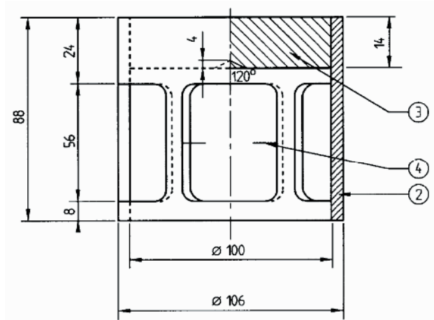
Fig. 1: Klockformig belastningstyngd, vikt 2 220 g, upphängningsbar på bronskolven.
